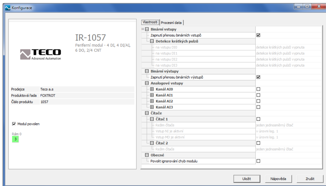
Obr.4.11 Konfigurace desky IR-1057
