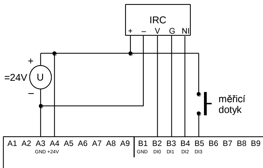
Obr.4.5 Příklad úplného připojení snímače polohy IRC
