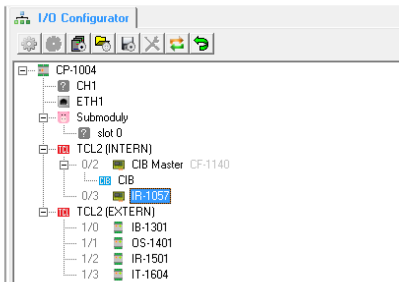
Obr.7.11 Sestava PLC CP-1004 s periferními moduly na sběrnici TCL2
