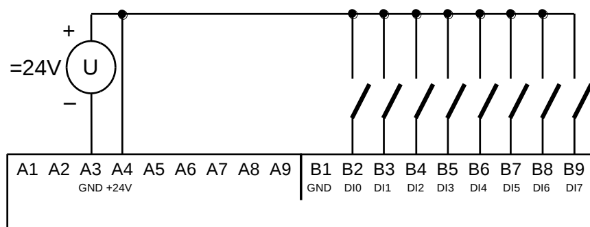
Obr.4.1 Typický příklad připojení spínačů k binárním vstupům základních modulů CP-10x4
