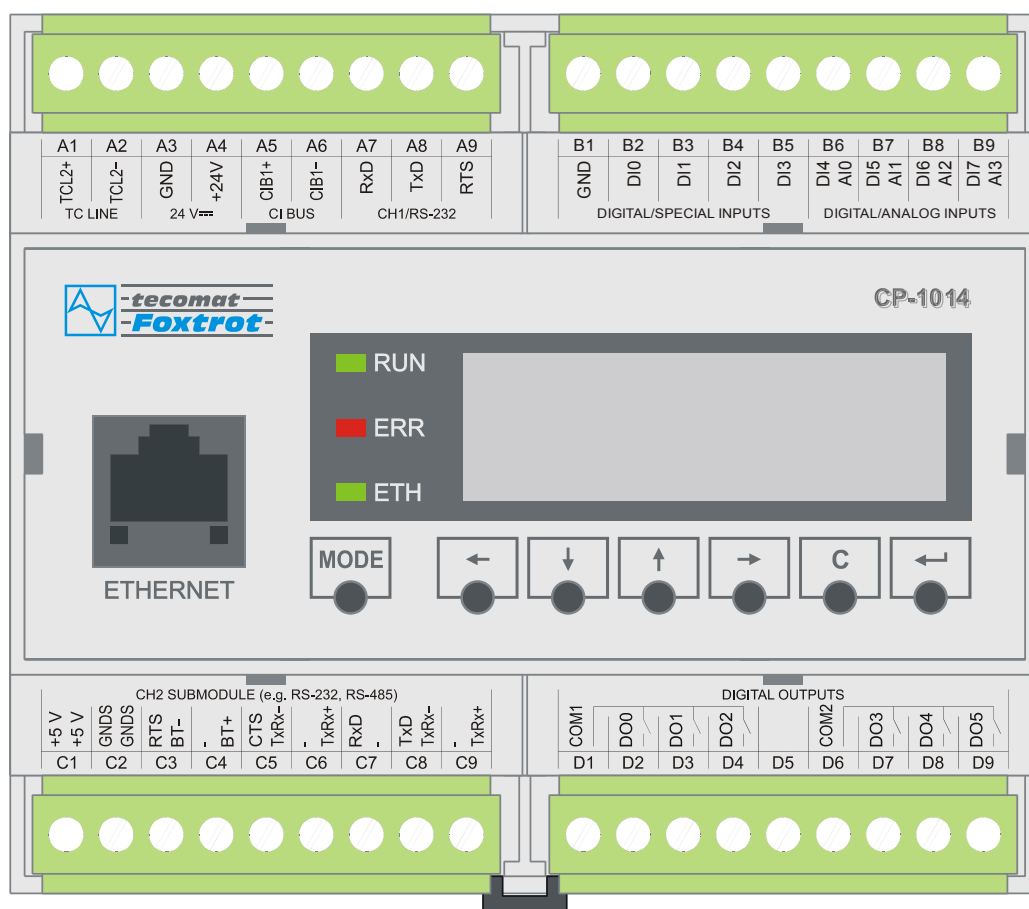
Obr.2.6 Základní modul CP-1014 - provedení od roku 2012
