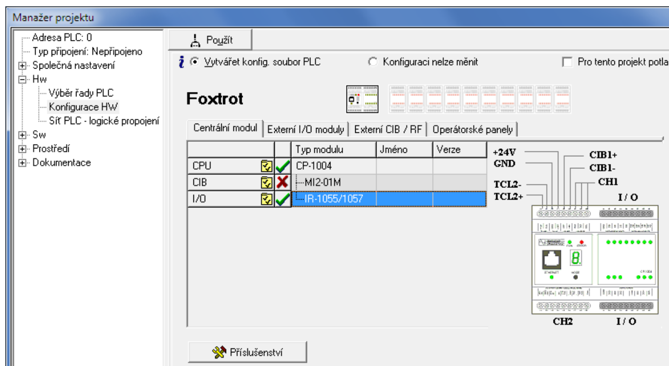
Obr.4.6 Konfigurace základního modulu CP-1004
