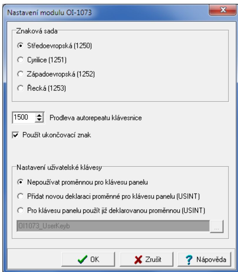
Obr.5.2 Konfigurace displeje OI-1083 (resp. OI-1073)
