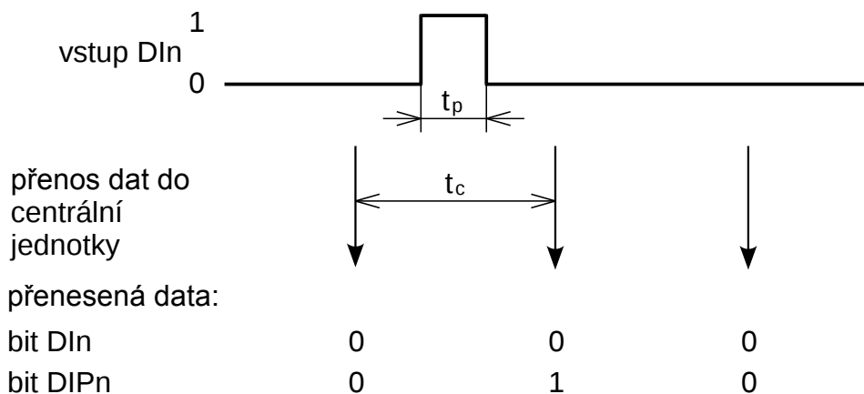
Obr.4.17 Funkce detekce krátkých pulzů do log.1 t_p - šířka pulzu, t_c = doba cyklu PLC
