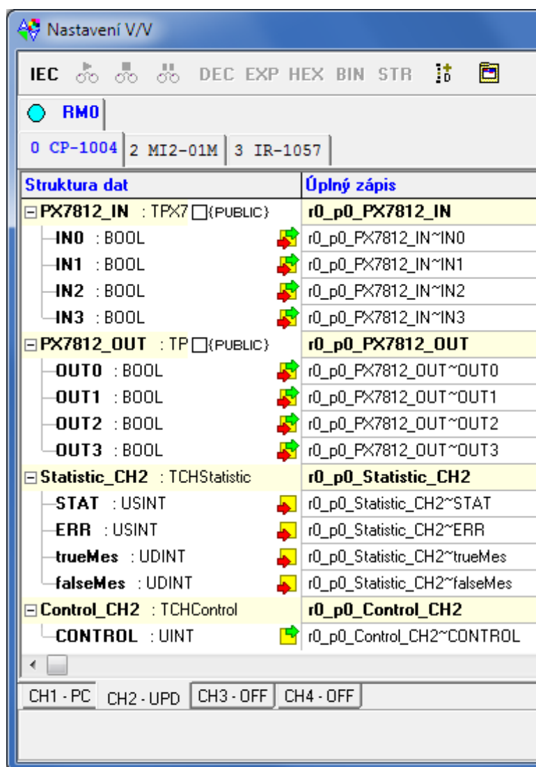
Obr.3.10 Struktura dat submodulu PX-7812
