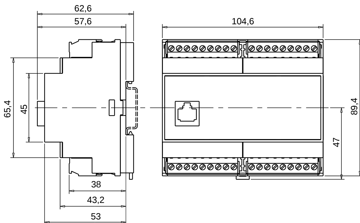
Obr.2.2 Rozměry základních modulů CP-10x4 v provedení s vyjímatelnými svorkovnicemi
