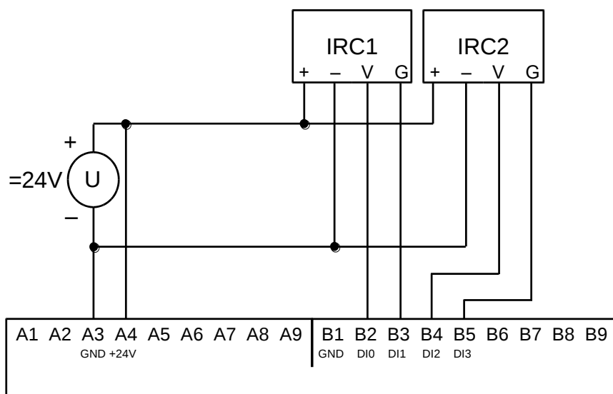
Obr.4.4 Příklad připojení dvou snímačů polohy IRC
