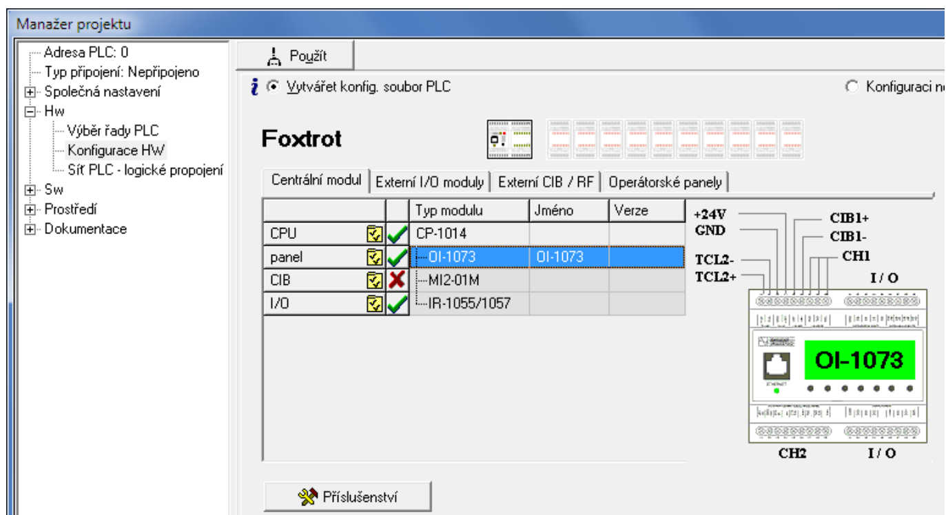
Obr.5.1 Konfigurace základního modulu CP-1014
