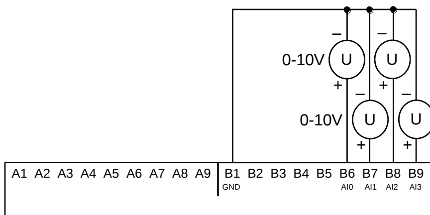
Obr.4.3 Typický příklad připojení signálů k analogovým vstupům základních modulů CP-10x4
