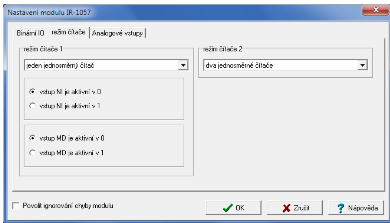
Obr.4.9 Konfigurace čítačů
