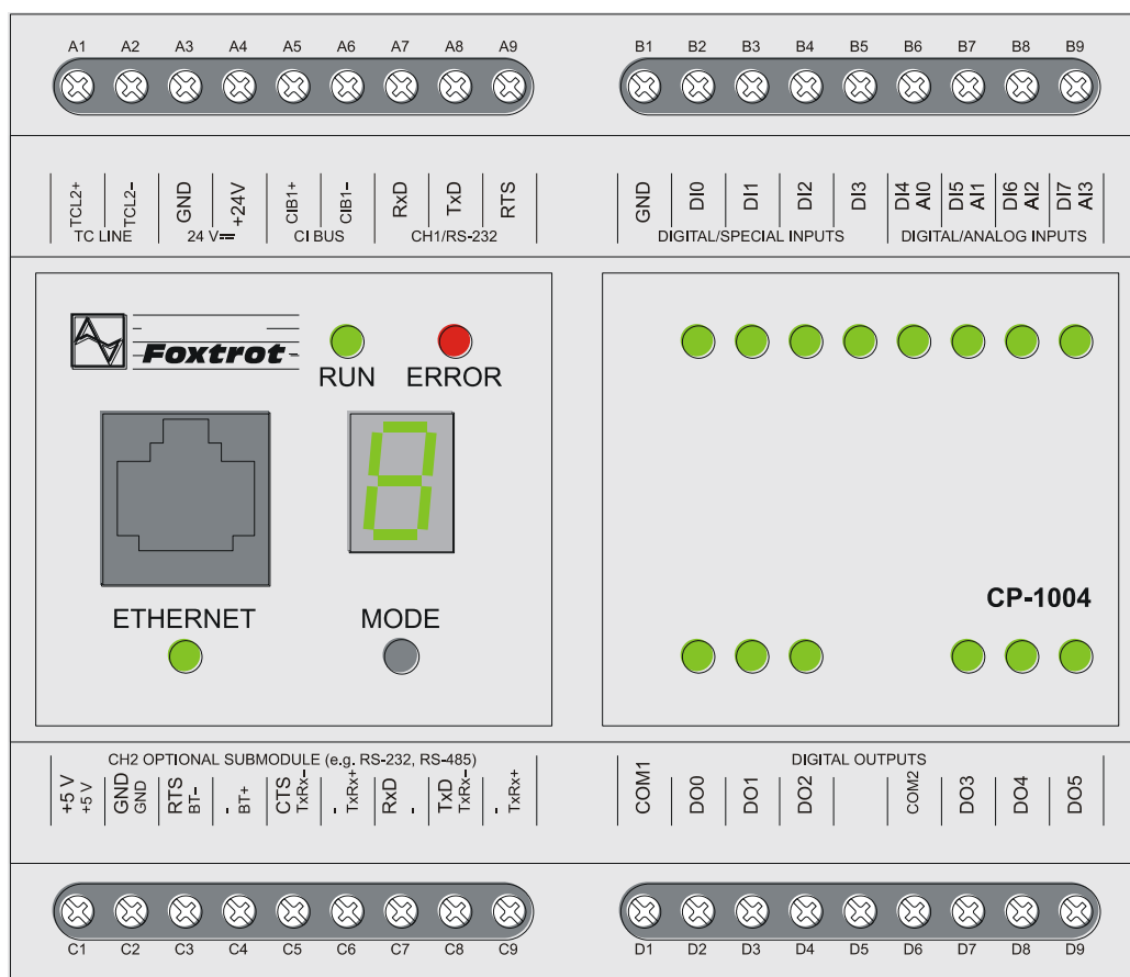
Obr.2.3 Základní modul CP-1004 - provedení do roku 2011
