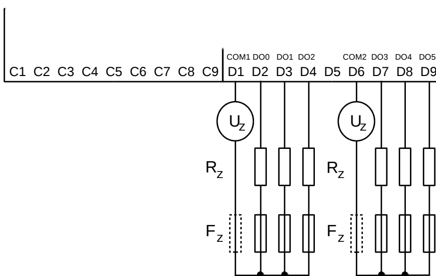
Obr.4.2 Typický příklad připojení zátěží k reléovým výstupům základních modulů CP-10x4
