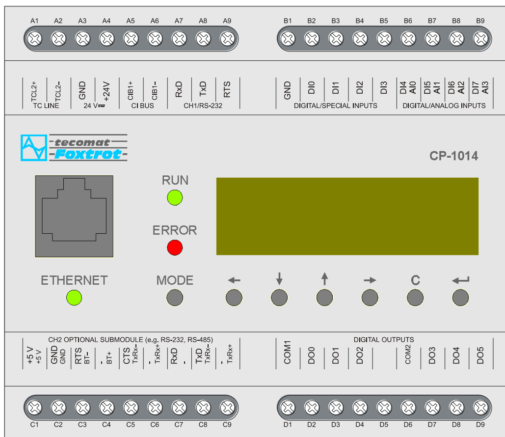
Obr.2.5 Základní modul CP-1014 - provedení do roku 2012
