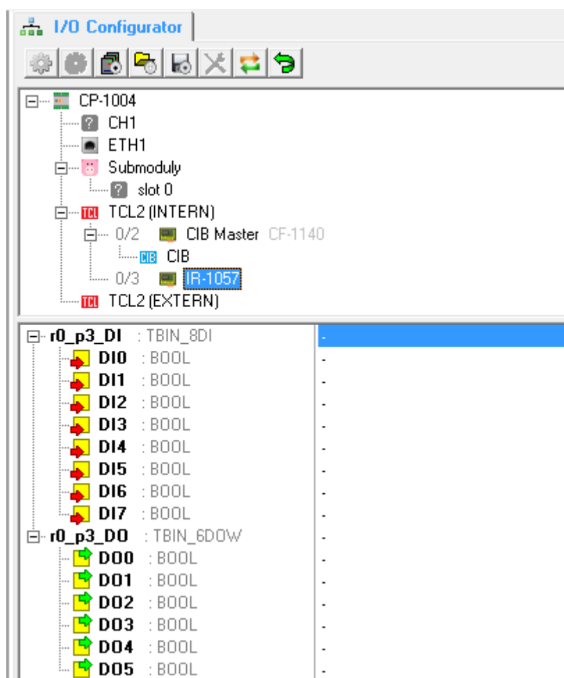
Obr.4.10 Okna nástroje I/O Configurator
