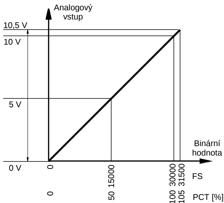
Obr.4.18 Napěťový rozsah analogových vstupů modulů CP-10x4
