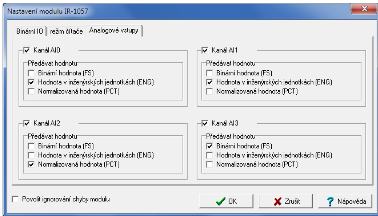
Obr.4.8 Konfigurace analogových vstupů
