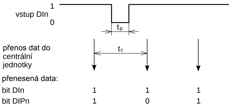
Obr.4.16 Funkce detekce krátkých pulzů do log.0 t_p - šířka pulzu, t_c = doba cyklu PLC
