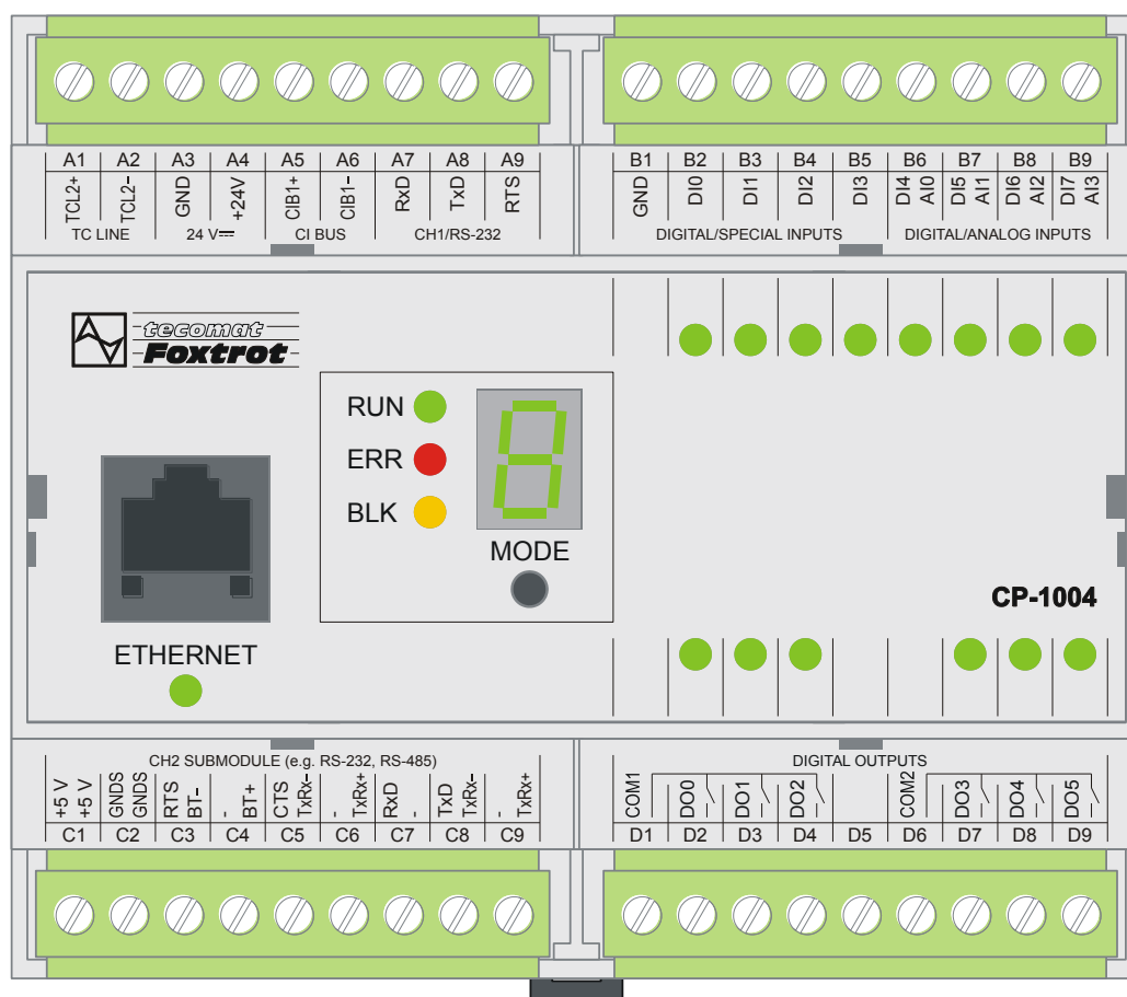
Obr.2.4 Základní modul CP-1004 - provedení od roku 2011
