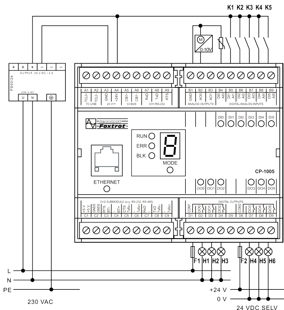
Obr. 4.1 Základní zapojení modulu CP-1005
